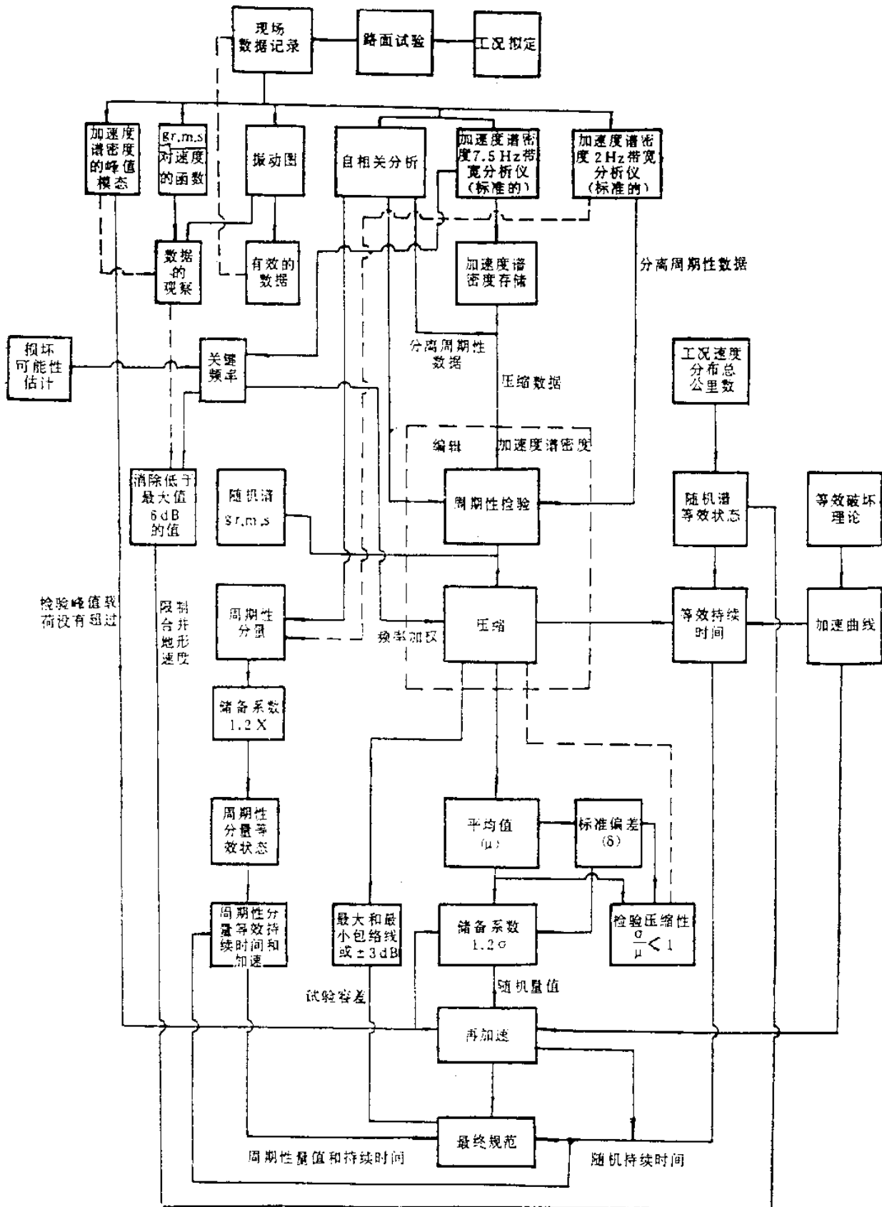
图 B1 振动试验条件的制订
